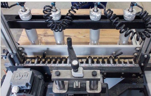
Dübelbohrmaschine
